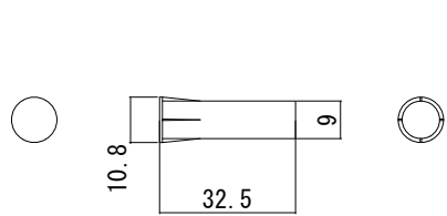
埋込型マグネット
