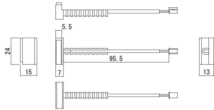
露出型マグネット
