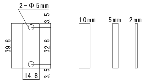
露出型マグネットスペーサー
