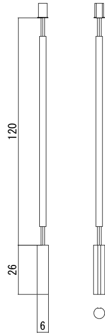
埋込型オートロックセンサー
